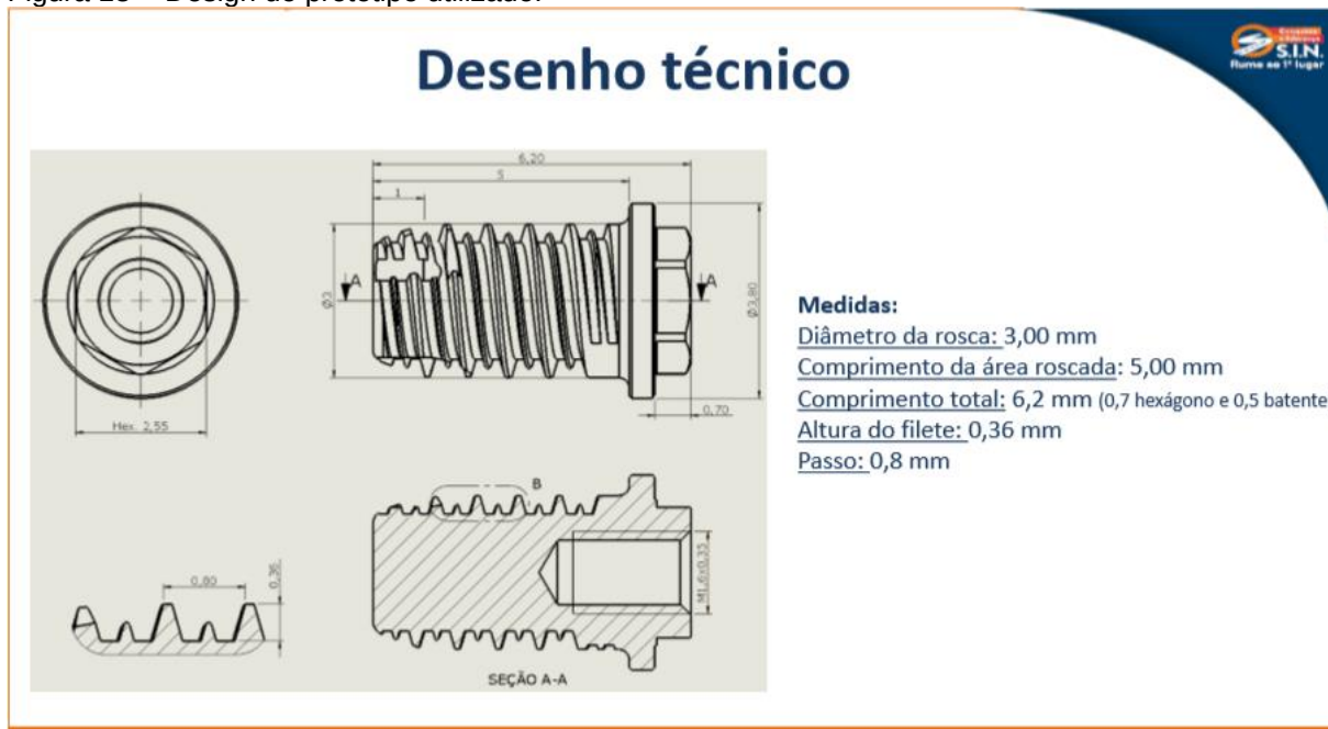
Figura 13 - Design do protótipo utilizado.
